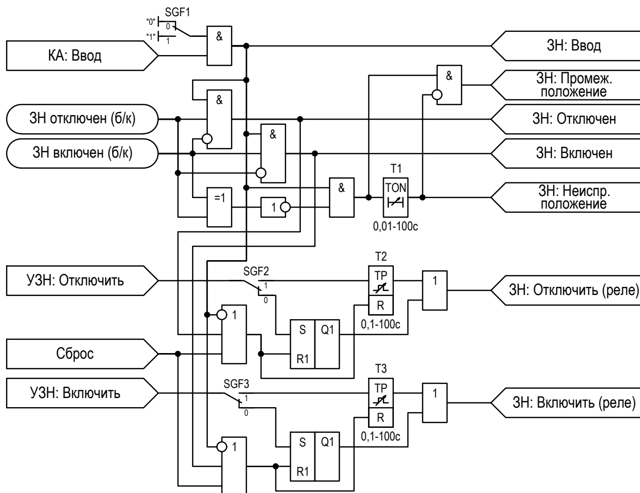
Рисунок 2.66 – Функциональная схема «ЗН»
